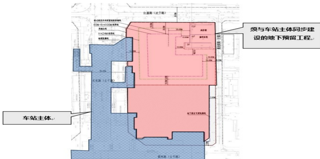
轨道交通车站及附属设施综合开发预留工程示意图
